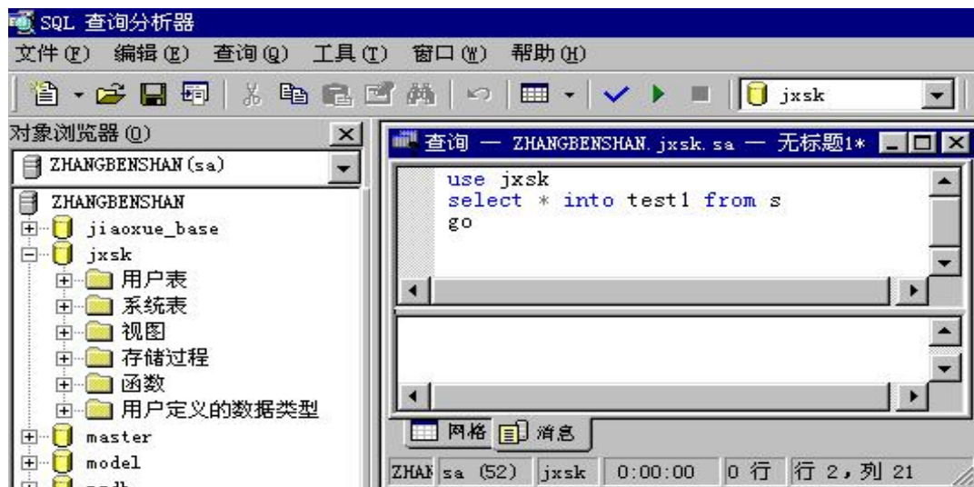
创建复制数据表SQL语句
